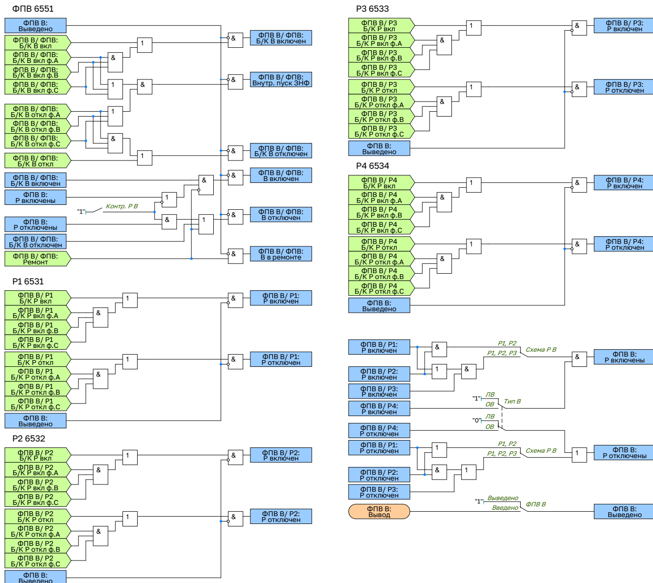
Рисунок 2.24 – Функциональная схема логики ФПВ В2
