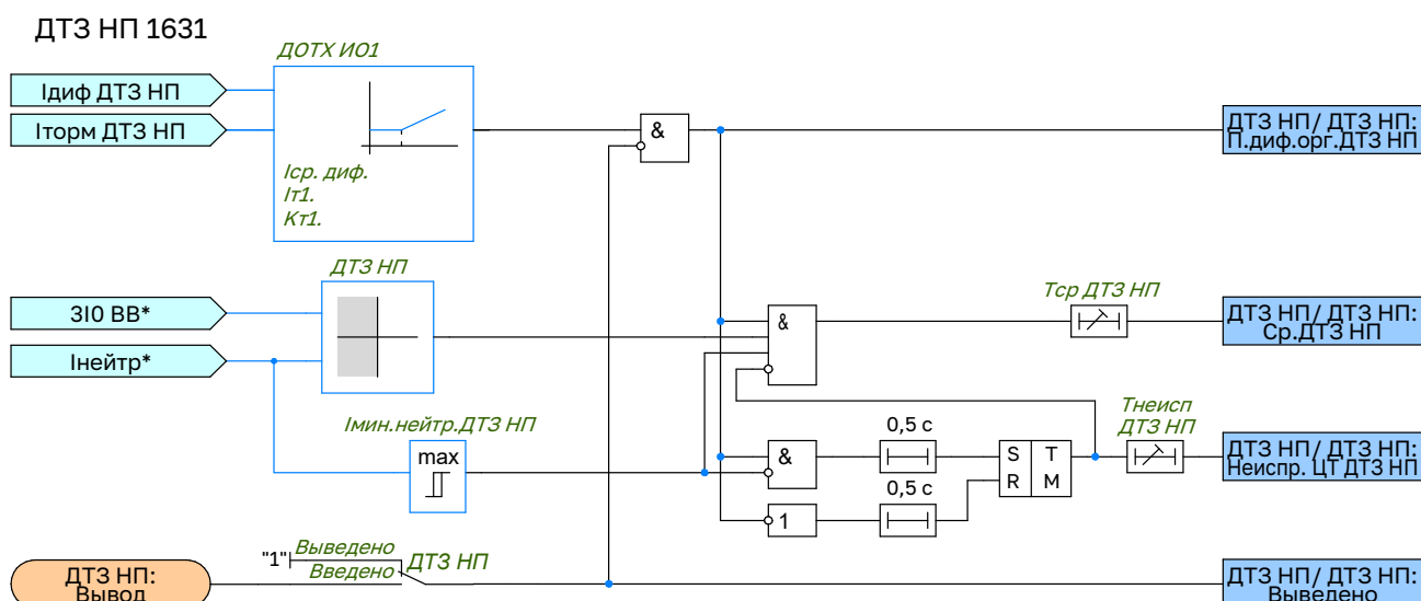
Рисунок 2.7 – Функциональная схема логики ДТЗ НП
